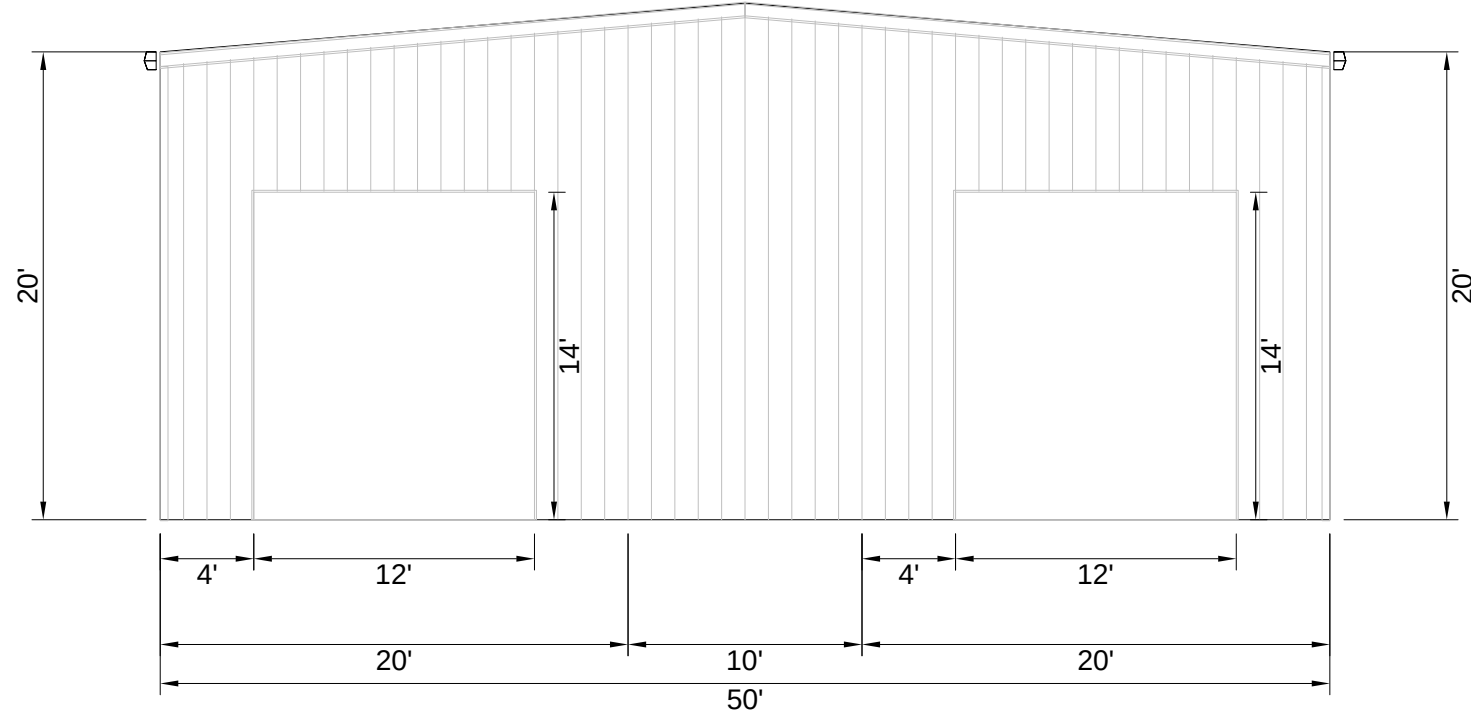
Left Wall
